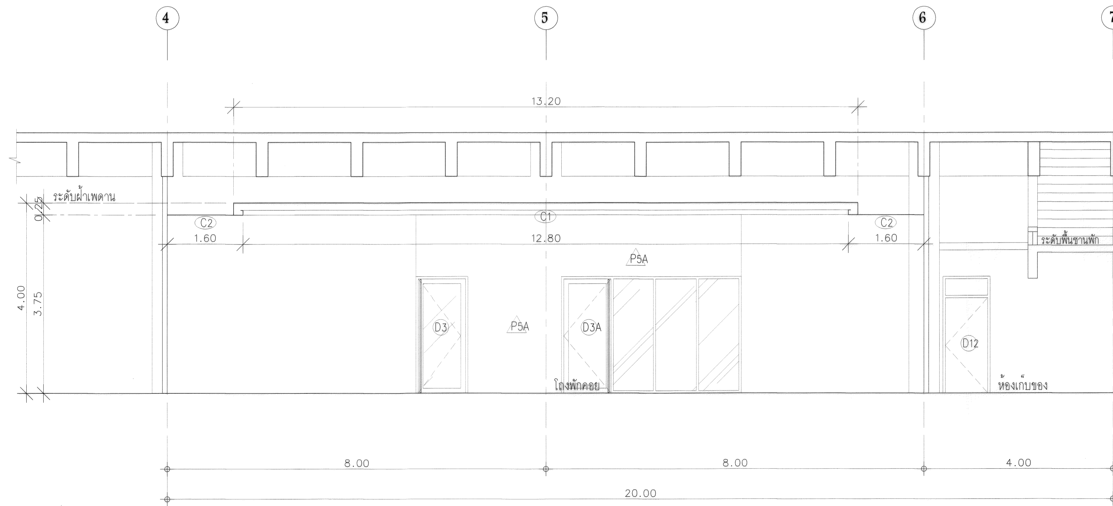
รูปตัด F 1:50 (หลังปรับปรุง)
