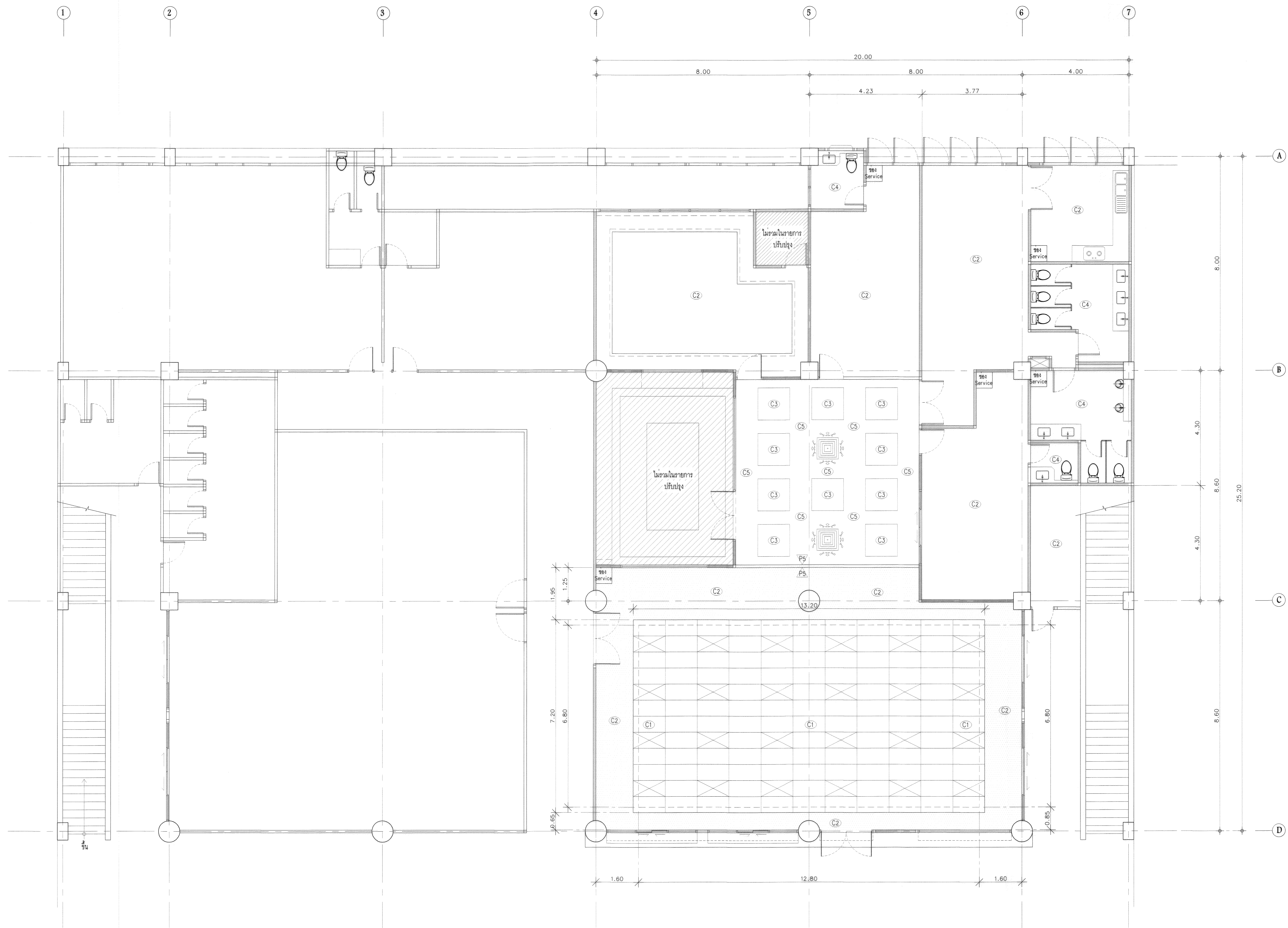
แปลน ฝ้าเพดาน 1:75 (หลังปรับปรุง)
