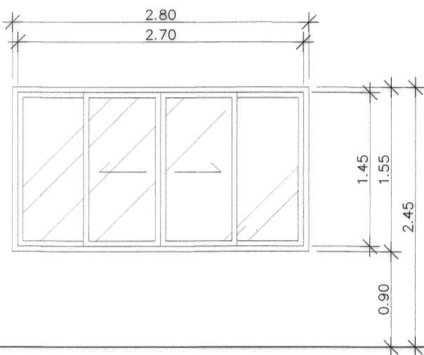
หน้าต่าง W2
