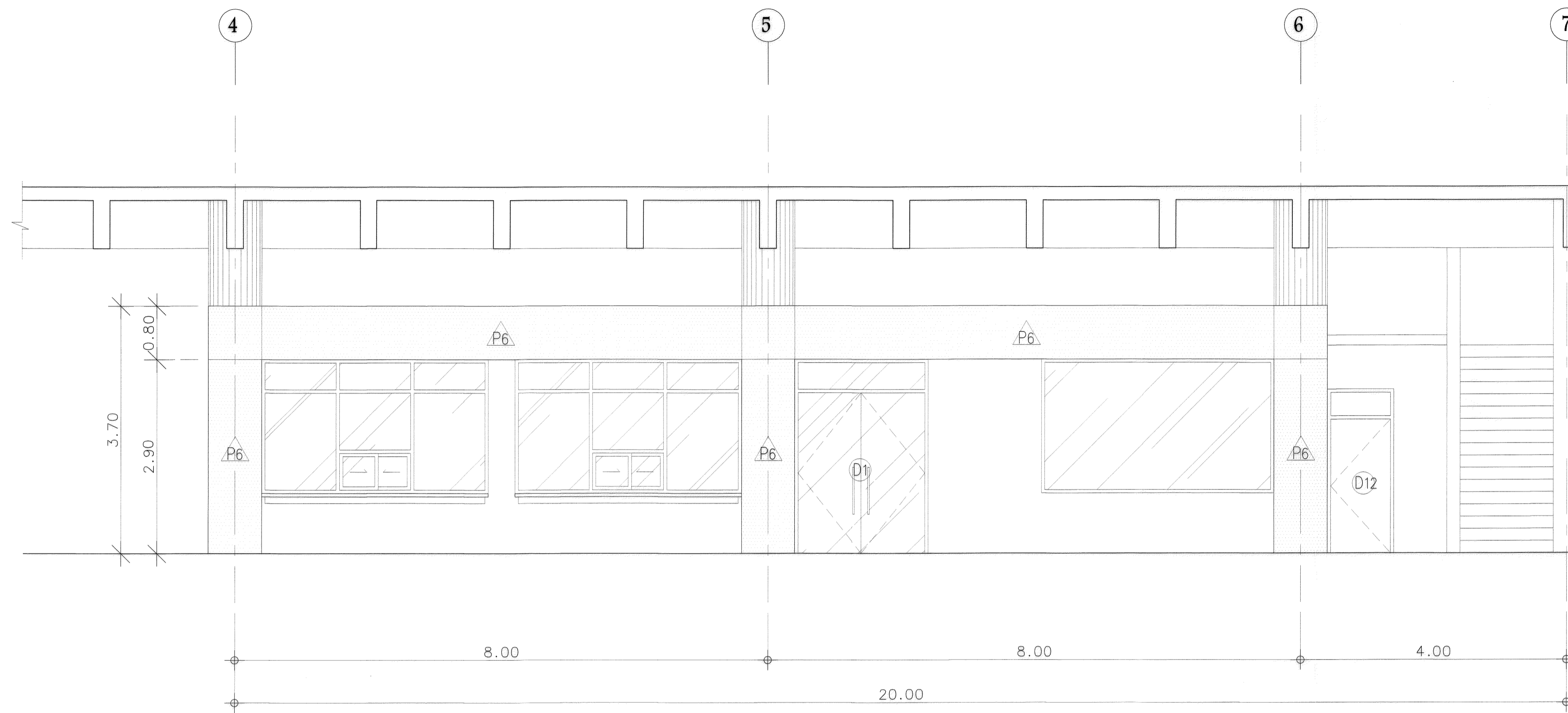
รูปตัด G 1:50 (หลังปรับปรุง)
