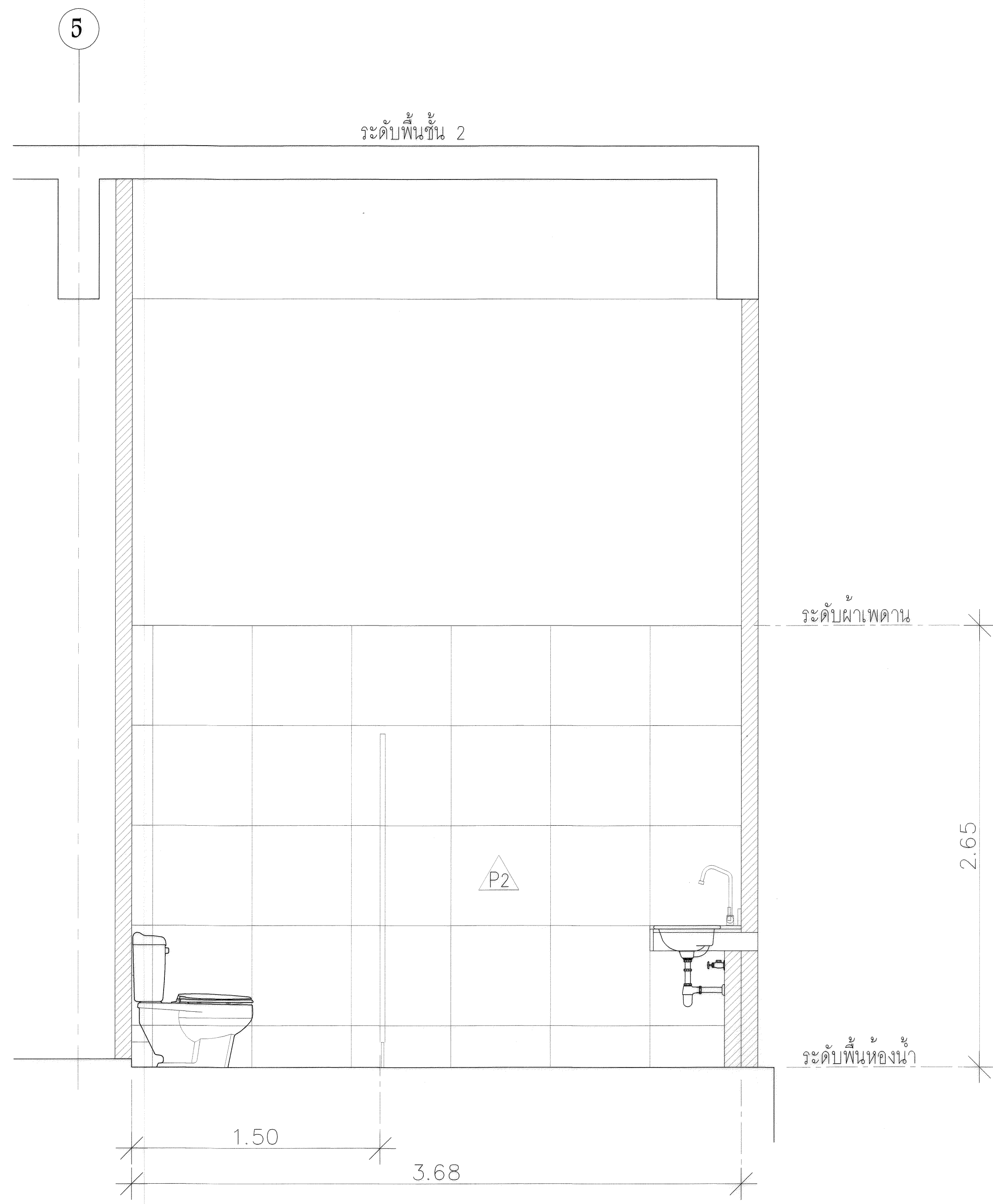
รูปตัด C 1:25
