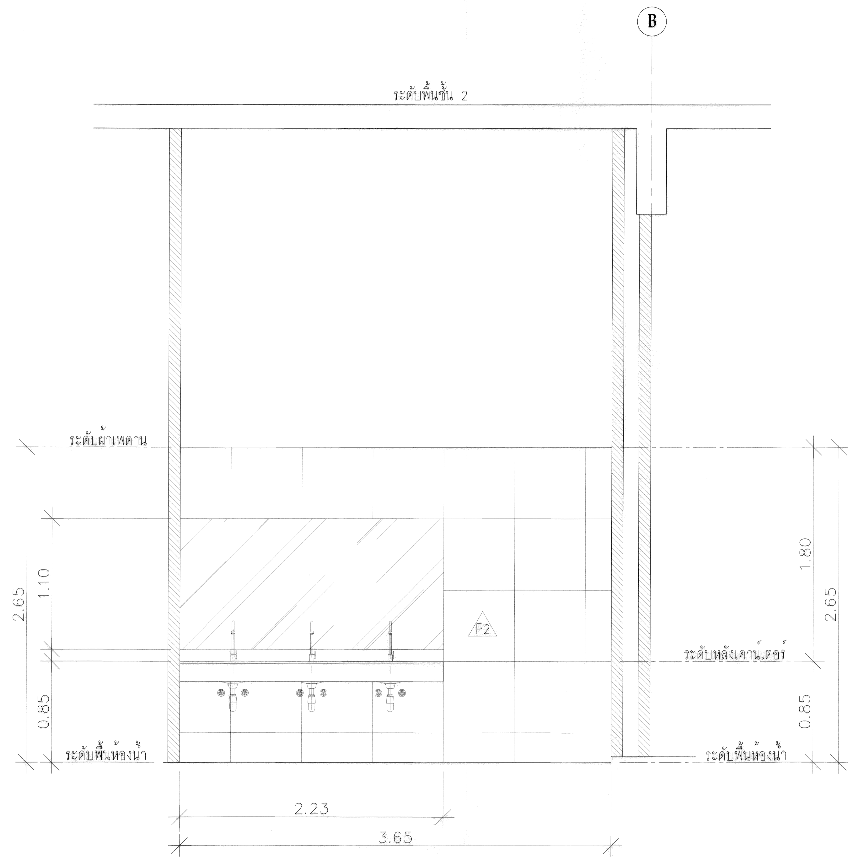
รูปตัด B 1:25
