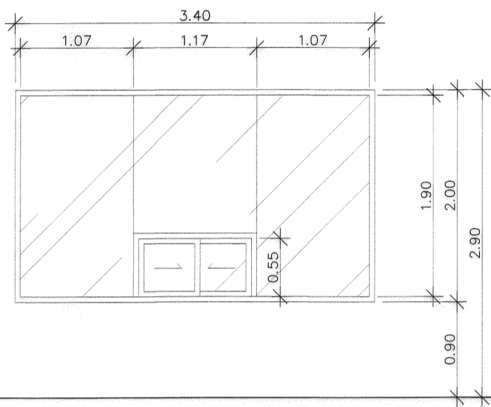
หน้าต่าง W3
