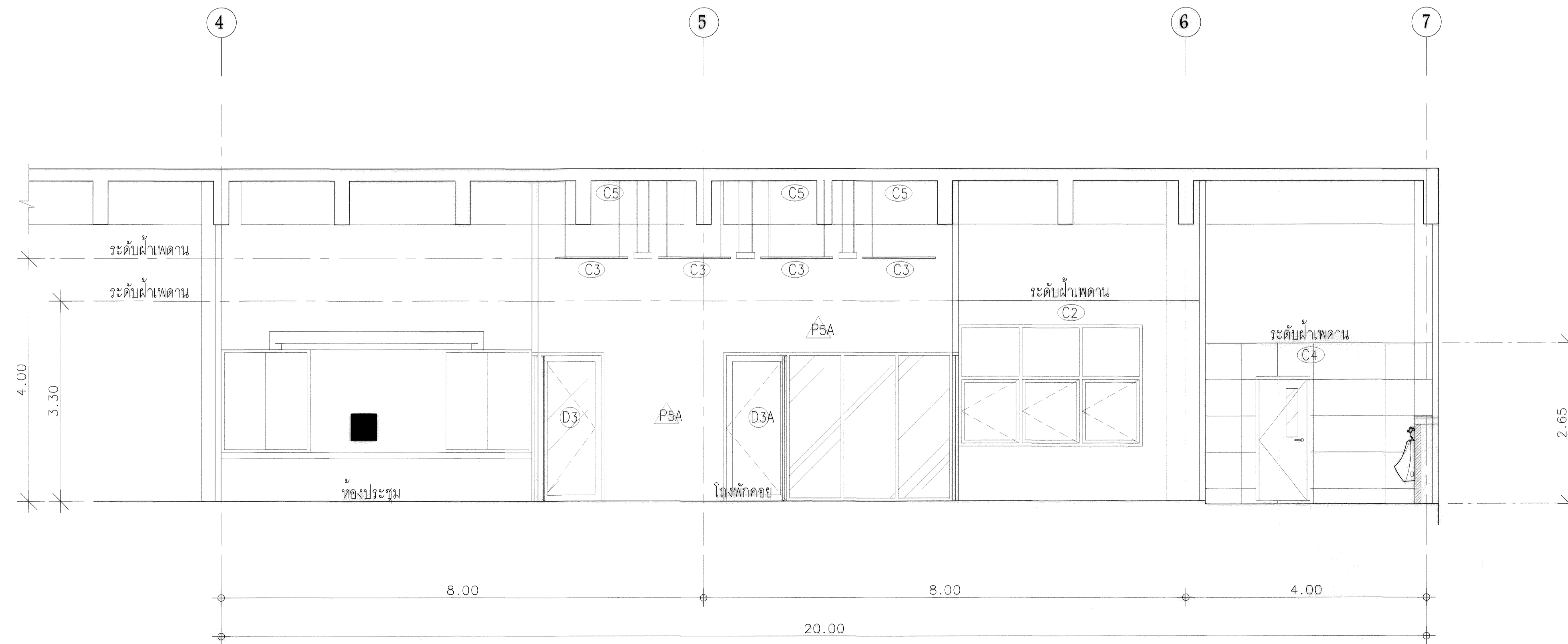
รูปตัด D 1:50 (หลังปรับปรุง)
