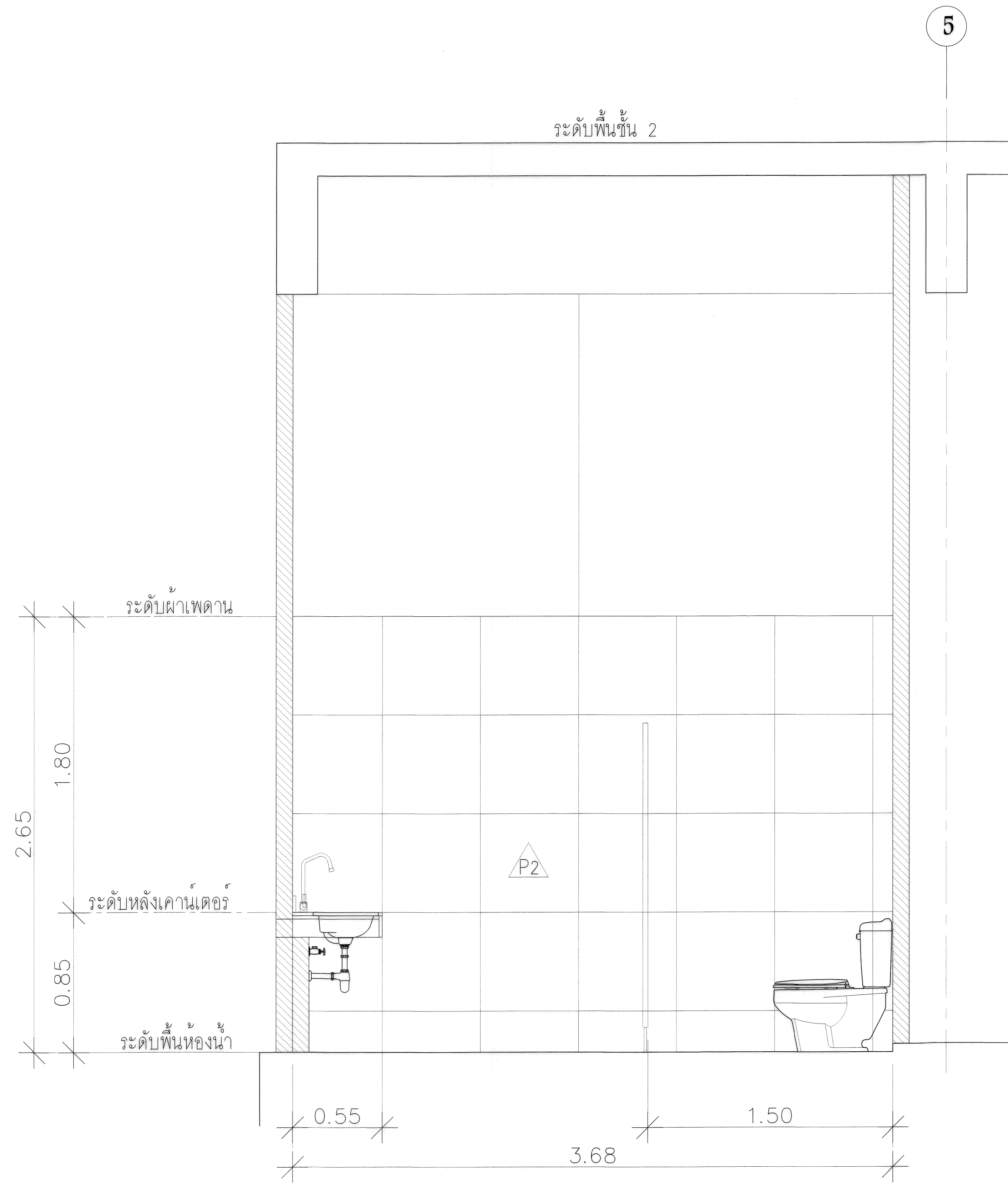
รูปตัด D 1:25
