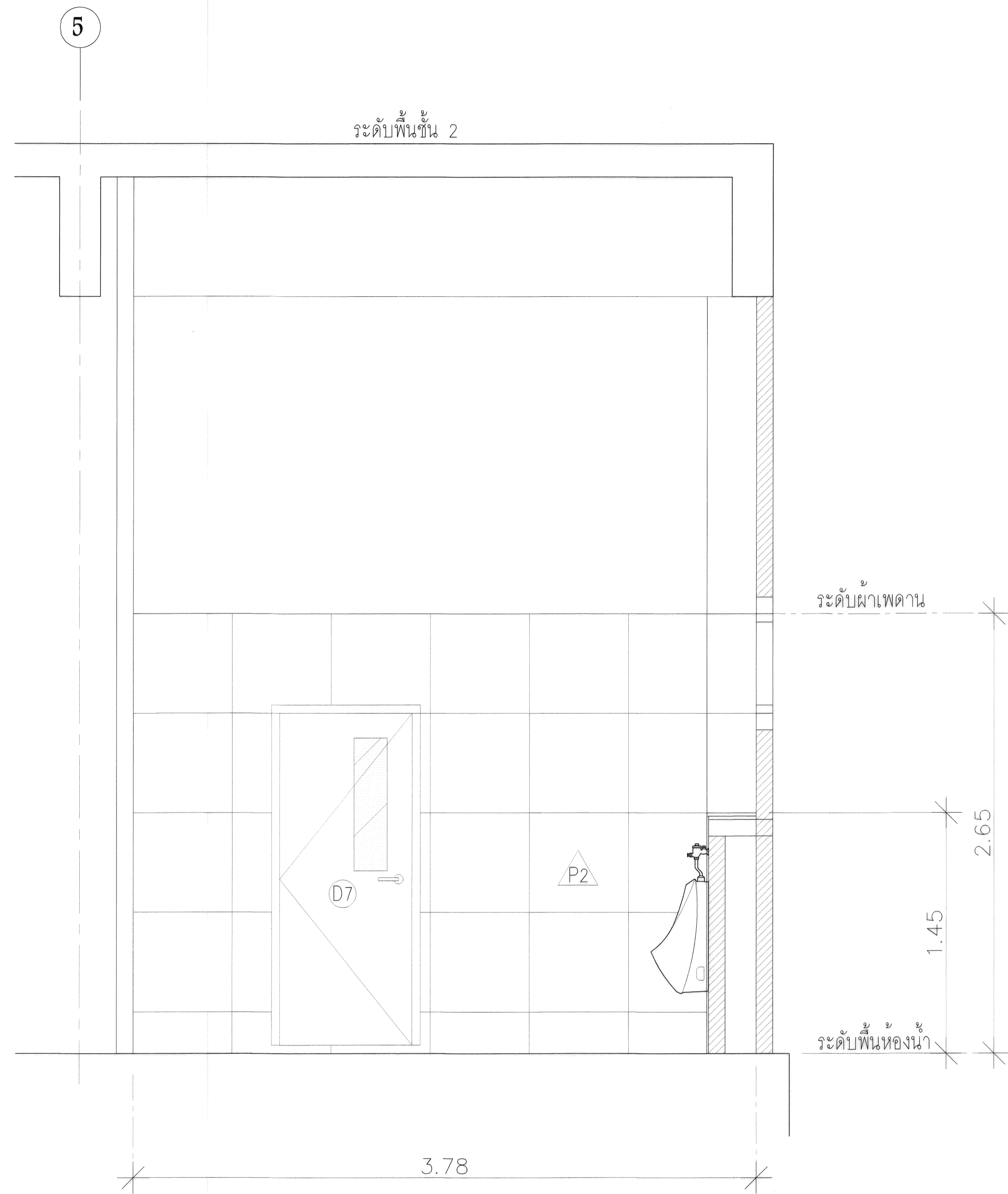
รูปตัด C 1:25
