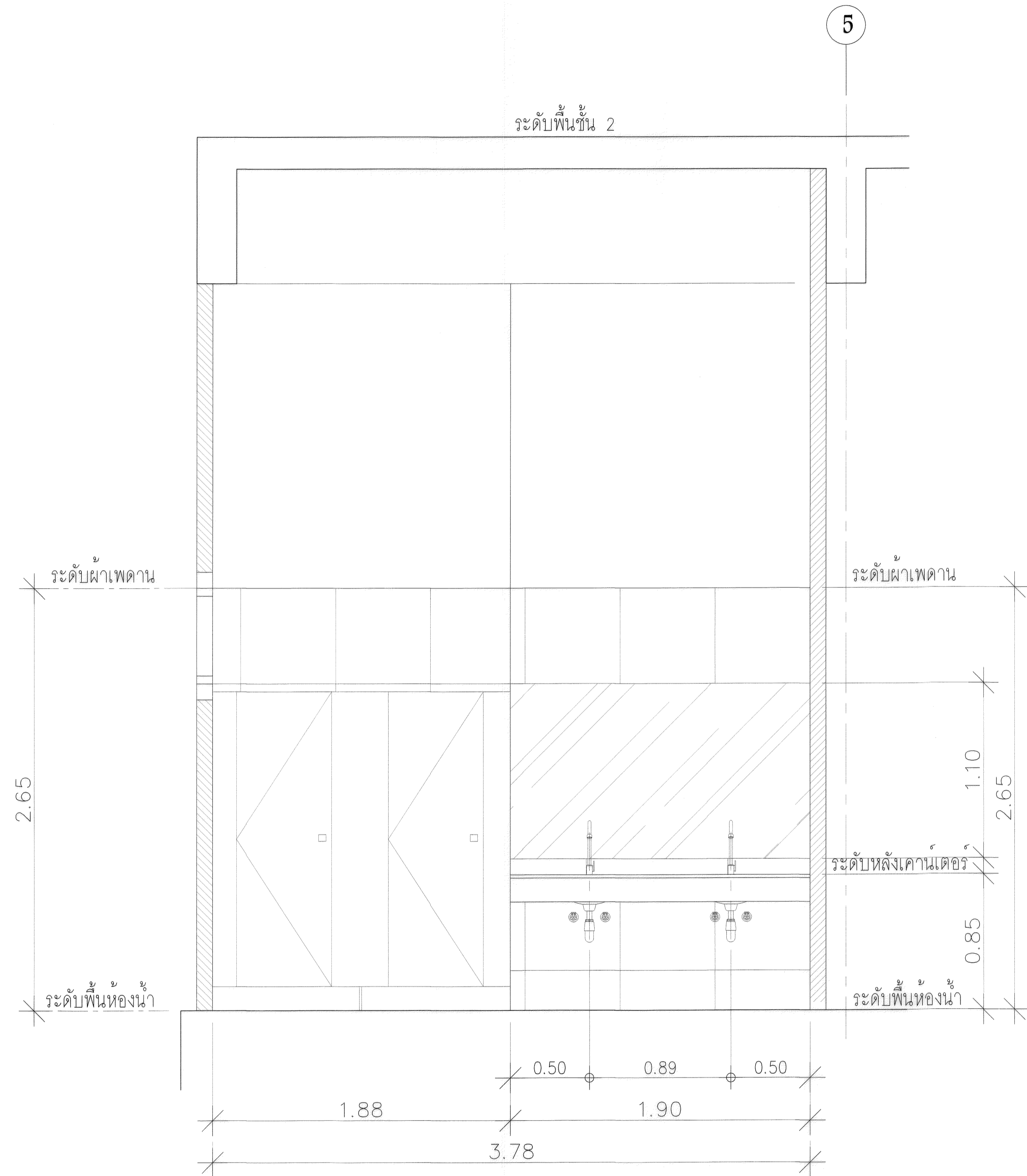
รูปตัด D 1:25
