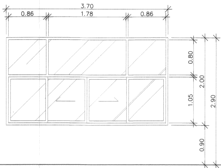
หน้าต่าง W1
