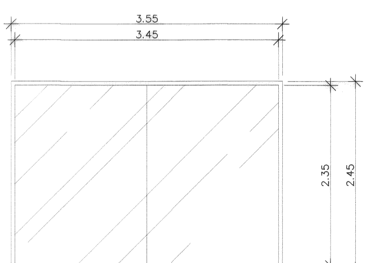
หน้าต่าง W4
