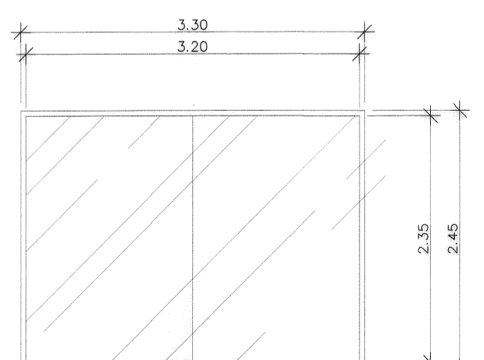
หน้าต่าง W5
