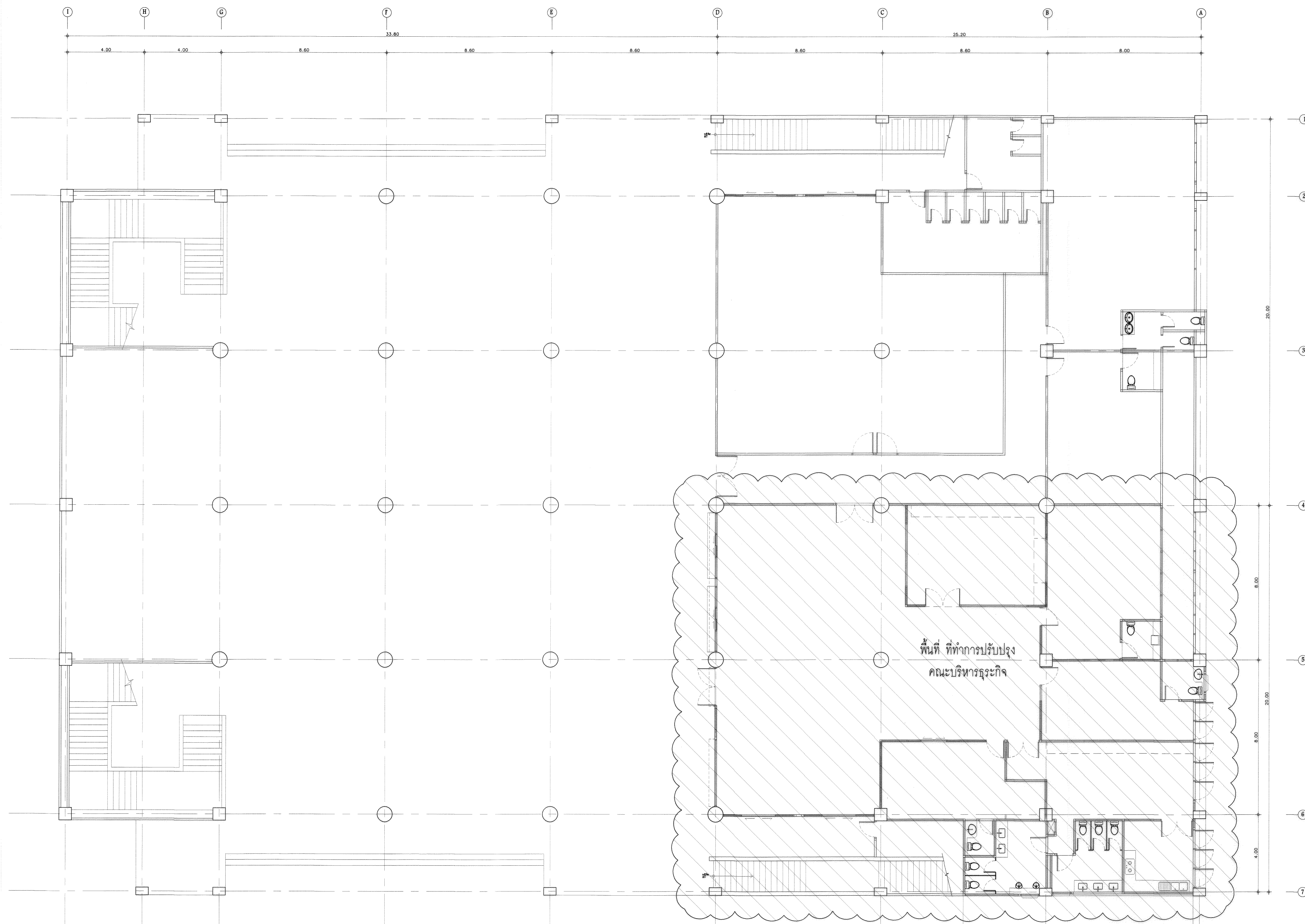
แปลน ชั้นกลาง 1:125 (หลังปรับปรุง)
