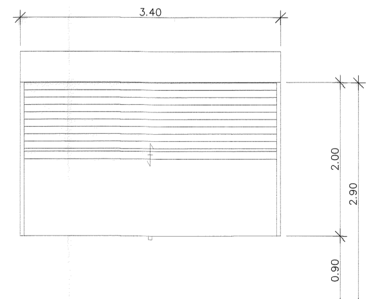
หน้าต่าง W3A
